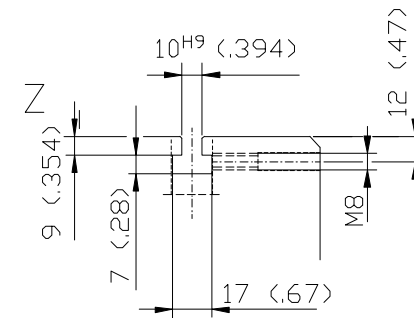
Ausschnitt Detail
