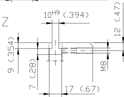
Ausschnitt Detail
